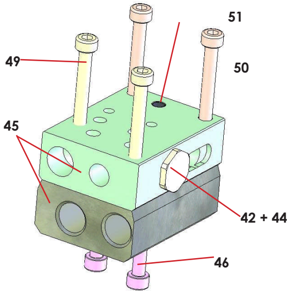
AVX (T) 129-690-080
