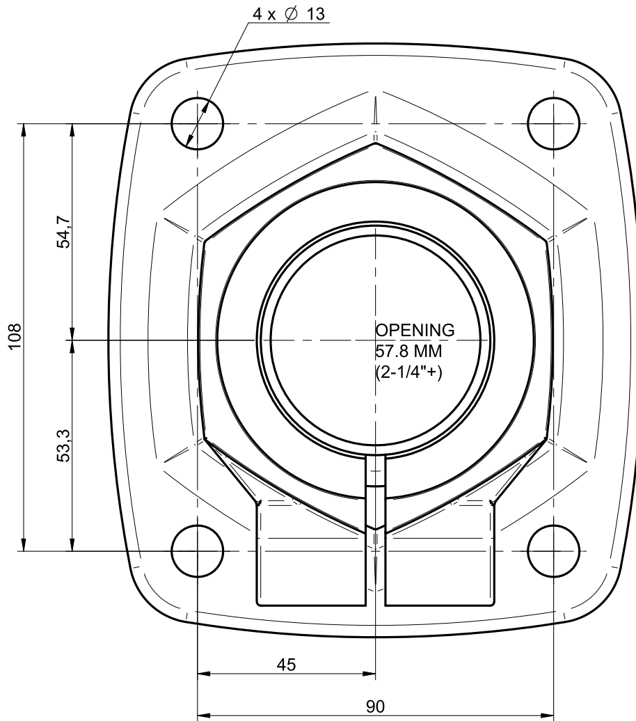
23200010 GRUPPO BASE TOP VIEW 187 MM TALL (7-3/8")
