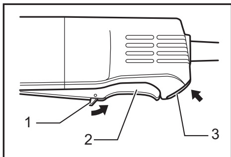
► 1. Palanca de desbloqueo 2. Palanca interruptora 3. Botón de bloqueo
