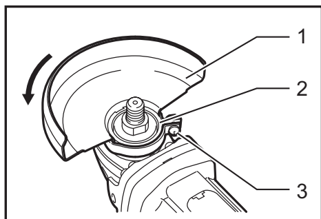
► 1. Protector (guarda) de disco 2. Caja de cojinetes 3. Tornillo
