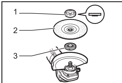
► 1. Contratuercas 2. Disco de centro hundido/multidisco 3. Brida interior
