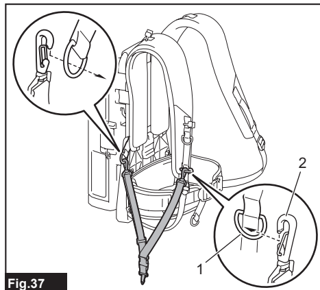
► 1. Anillo 2. Gancho
