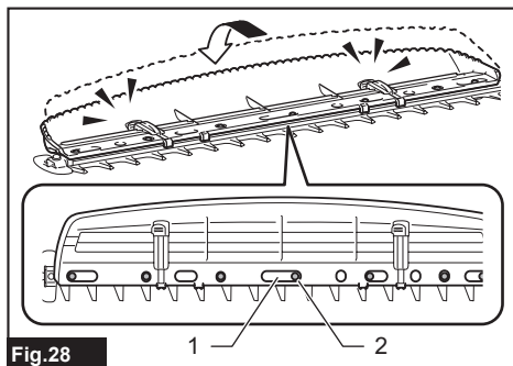
► 1. Hole 2. Screw
