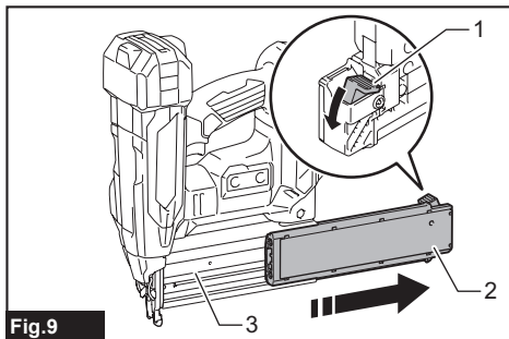
► 1. Lever 2. Slide door 3. Magazine
