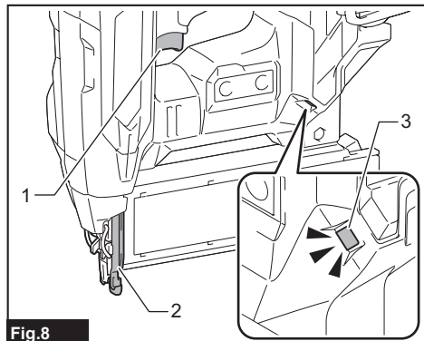
► 1. Switch trigger 2. Contact element 3. Lamp
